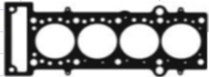
41103 SC - 1,2 MM - CIL. 78 MM 41103 MLS - 0,7 MM - CIL. 78 MM 41103 MLS-1M - 1,0 MM - CIL. 78 MM JTA CABEÇOTE
