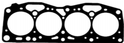
40501 SC - 1,9 MM - CIL. 87 MM 40501 KT - 2,9 MM - CIL. 87 MM 40501 TB - 2,4 MM - CIL. 87MM
