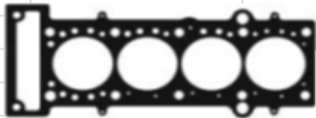
41102 SC - 1,2 MM - CIL. 82,2 MM 41102 MLS - 0,7 MM - CIL. 82,2 MM 41102-MLS-1M - 1,0 MM - CIL. 82,2 MM JTA CABEÇOTE
