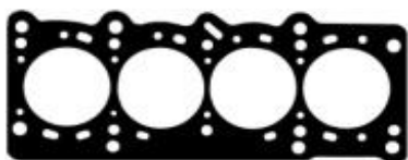
40101 SC - 1,2 MM - CIL. 71,5 MM 40101 MLS - 0,5 MM - CIL. 71,5 MM 40101 MLS-3M - 1,5 MM - CIL. 71,5 MM 40101 KT - 2,2 MM - CIL. 71,5 MM
