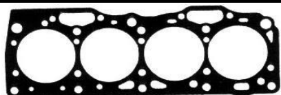
40601 SC - 1,9 MM - CIL. 87 MM 40601 KT - 2,9 MM - CIL. 87 MM 40601 TB - 2,4 MM - CIL. 87 MM JTA CABEÇOTE
