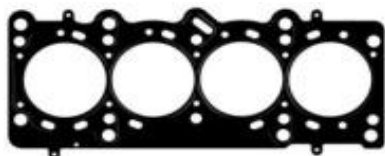
40103 SC - 1,2 MM - 72,5 MM 40103 MLS - 0,5 MM - 72,5 MM 40103 MLS-2M - 1,0 MM - CIL. 72,5 MM 40103 KT - 2,2 MM - CIL. 72,5 MM
